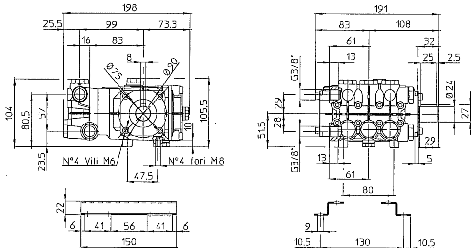
DIMENSIONI D'INGOMBRO POMPA ALBERO MASCHIO - DIMENSIONAL DRAWING PUMP WITH MALE SHAFT
