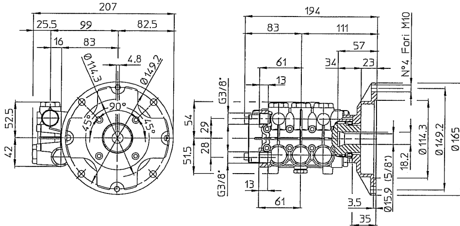
DIMENSIONI D'INGOMBRO POMPA ALBERO MASCHIO - DIMENSIONAL DRAWING PUMP WITH MALE SHAFT
