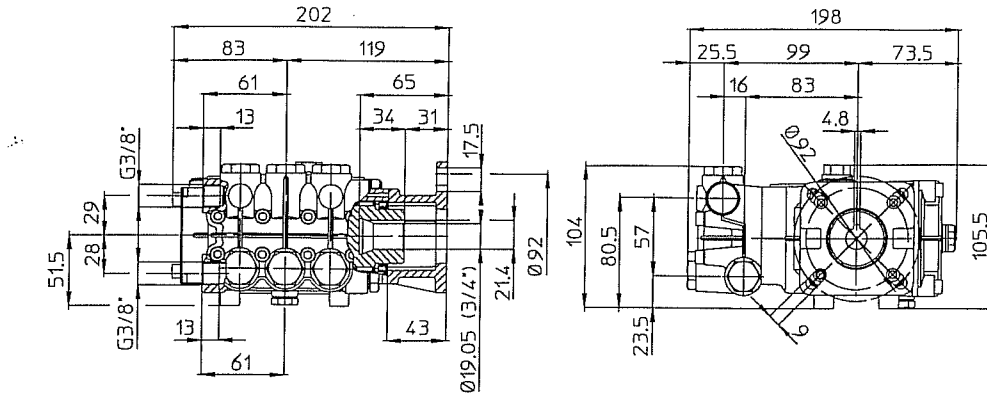
DIMENSIONI D'INGOMBRO POMPA FLANGIATA P03 - DIMENSIONAL DRAWING PUMP WITH FLANGE P03
